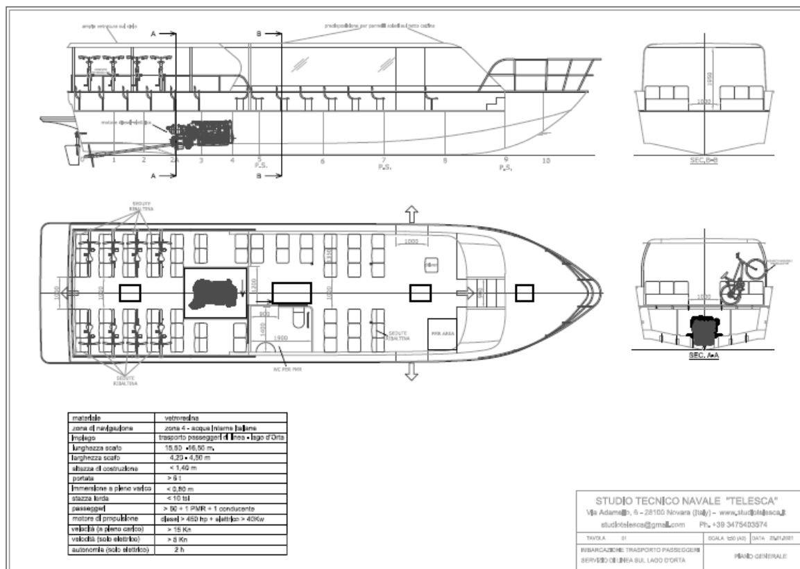
Figura 57 – Piano generale progetto nuova imbarcazione
