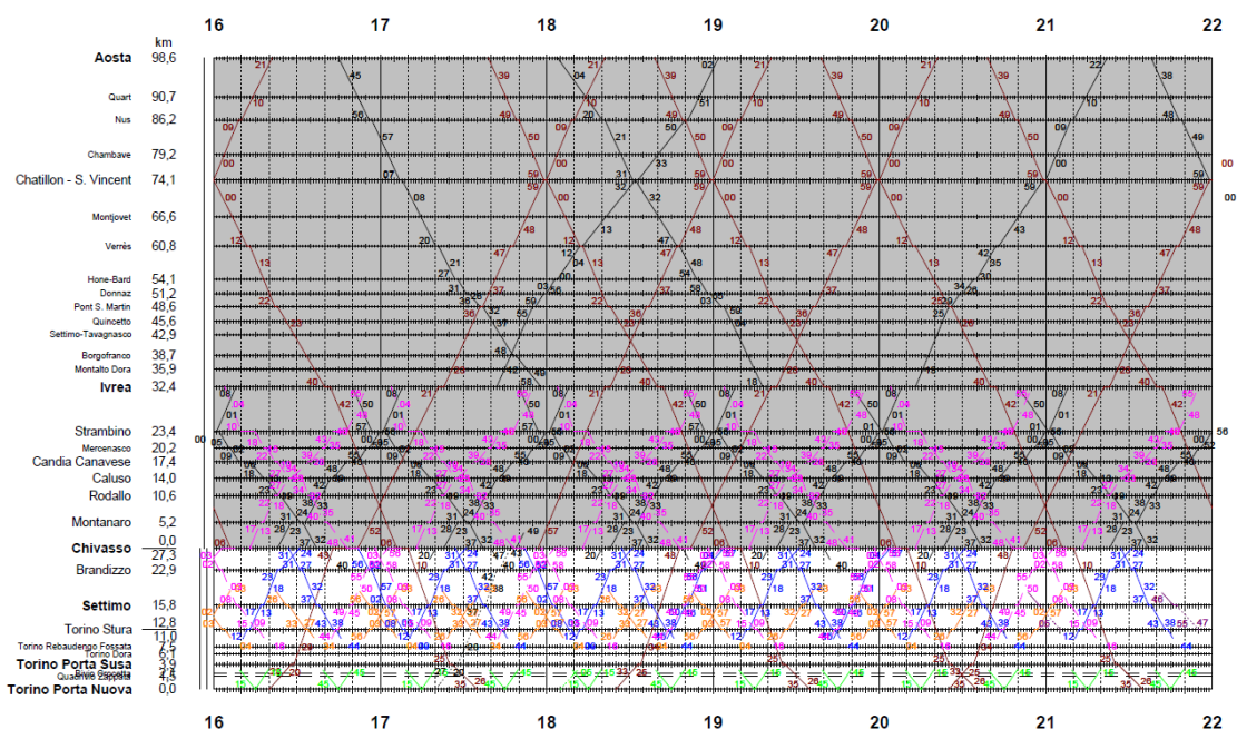
Figura 1 - Orario grafico del prolungamento linea sfm8 a Ivrea. In rosa la linea sfm8 sovrapposta al servizio attuale dei R Ivrea-Chivasso-Novara (in nero) e ai RV della Valle d'Aosta (in marrone)
