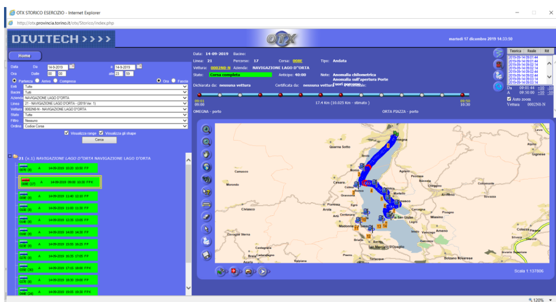
Figura 37 – Sistema di monitoraggio implementato sul Lago d'Orta.
